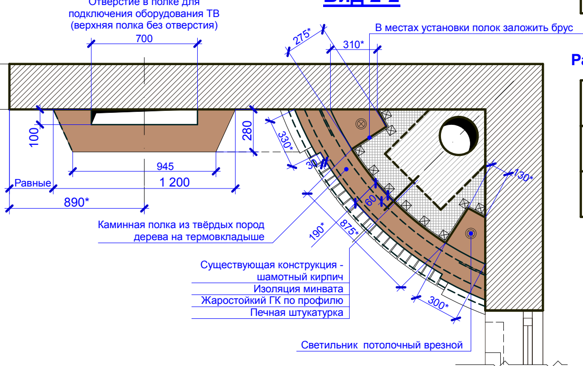
Вид 2-2
