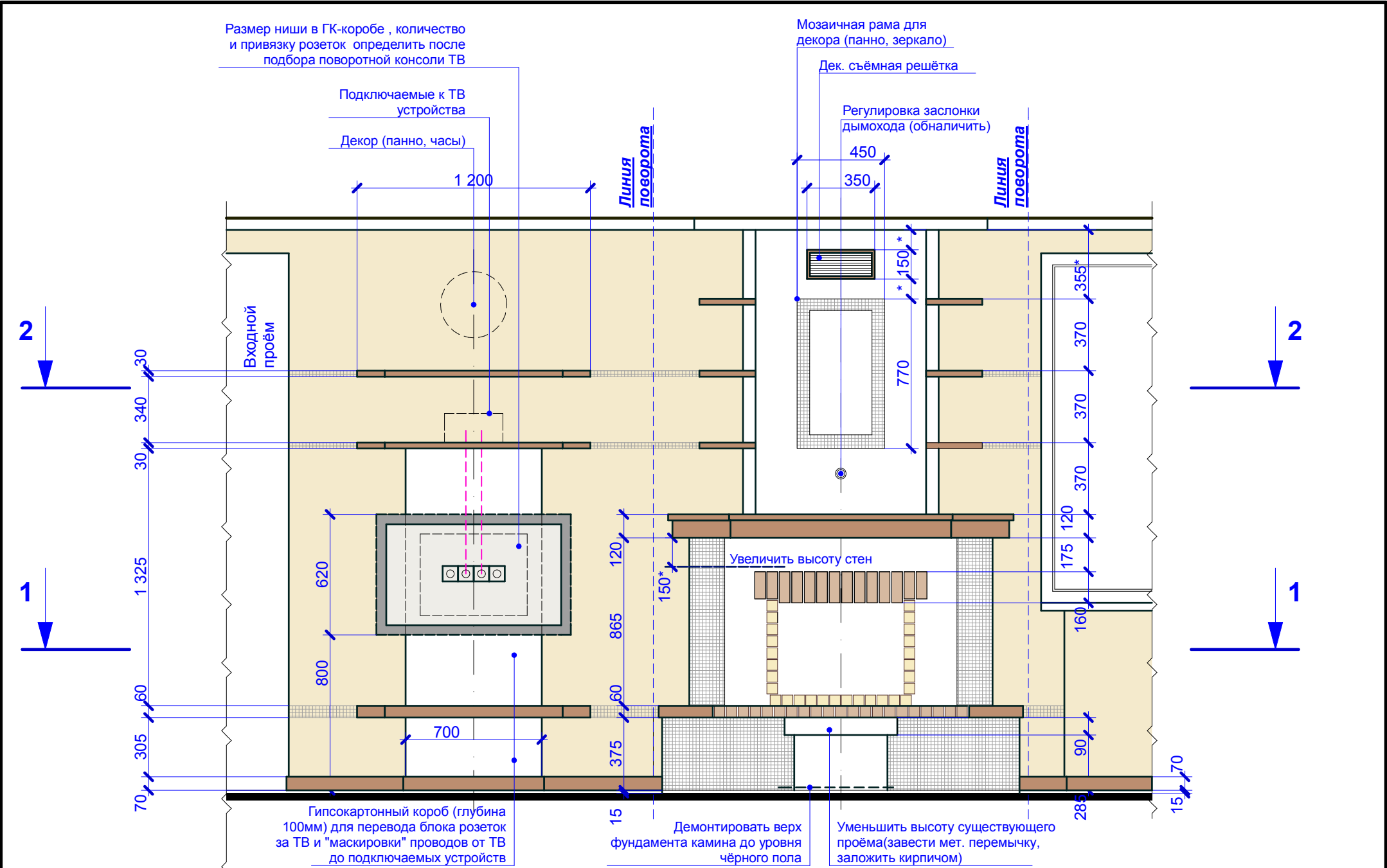
Вид 1-1
