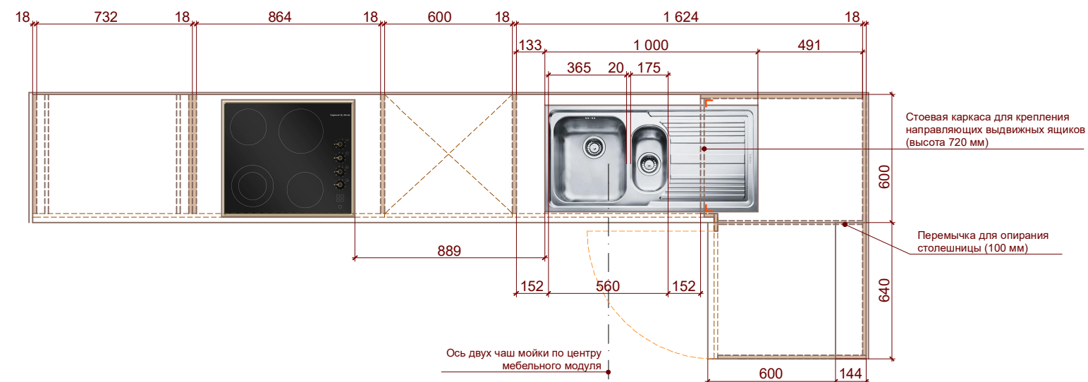
Схема размещения стоевых каркаса для опирания столешницы
