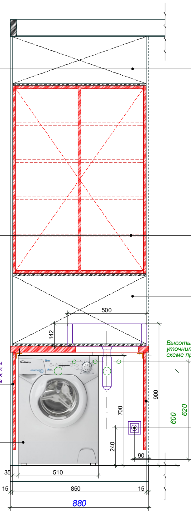
Сечение мебельного модуля по развёртке 3
