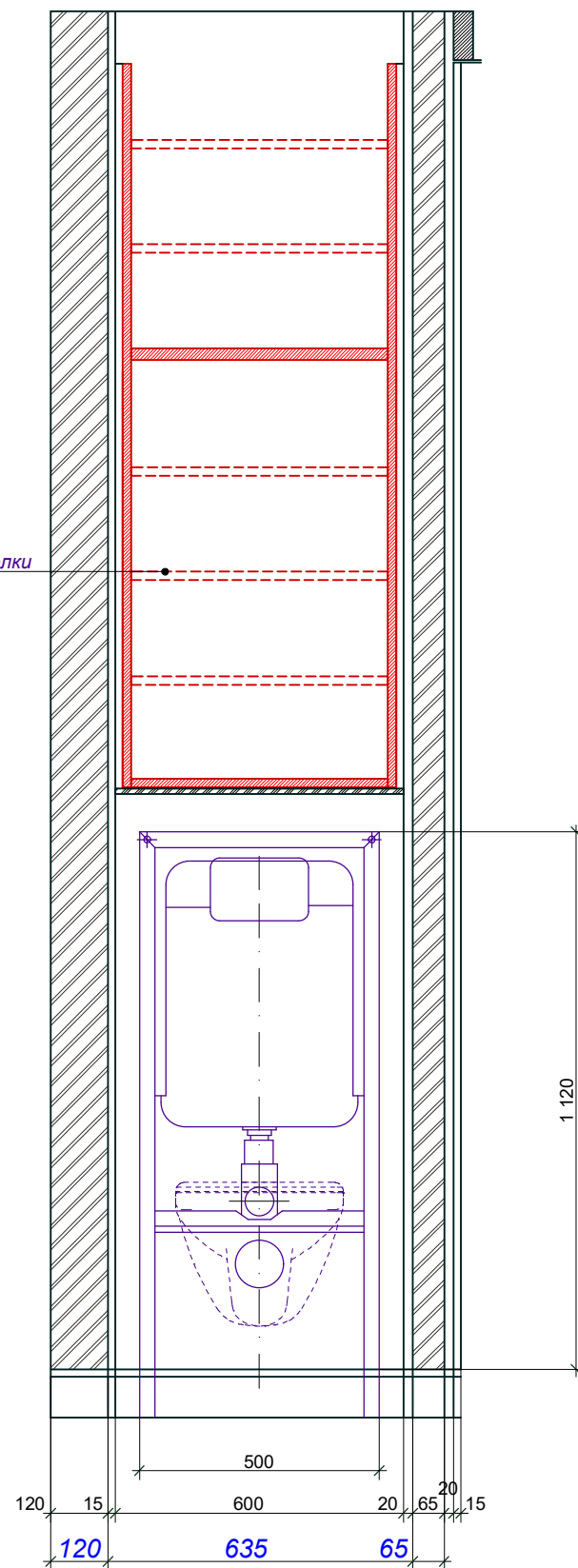
Сечение мебельного модуля по развёртке 5
