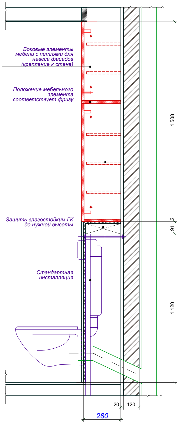
Сечение мебельного модуля по развёртке 4
