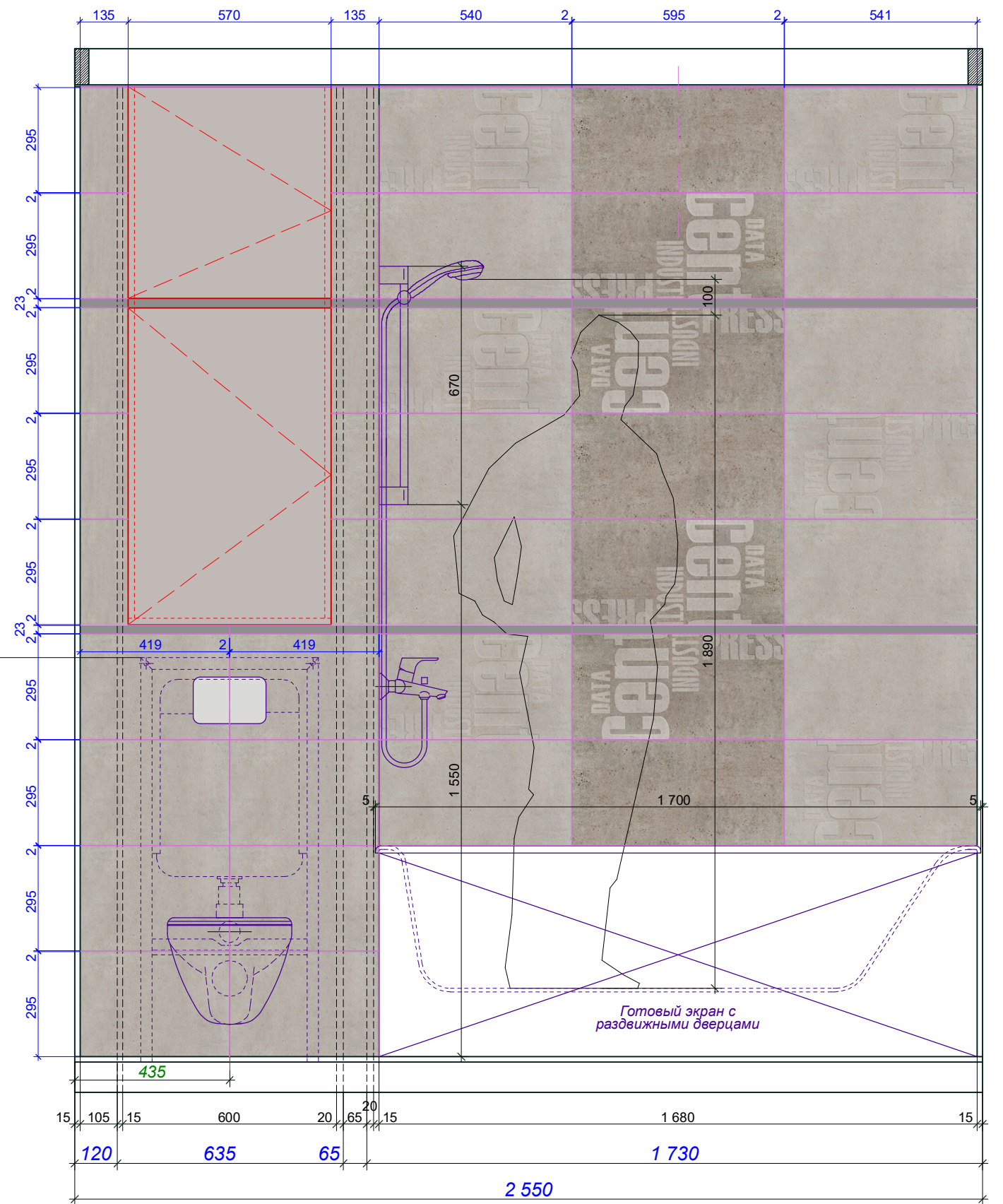
Развёртка 5
