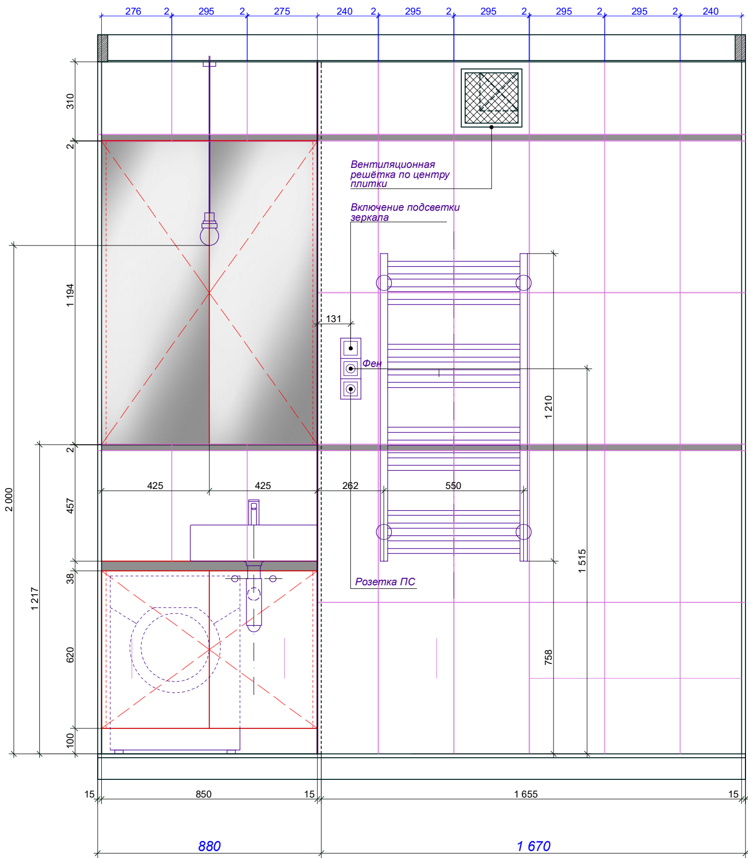
Развёртка 3
