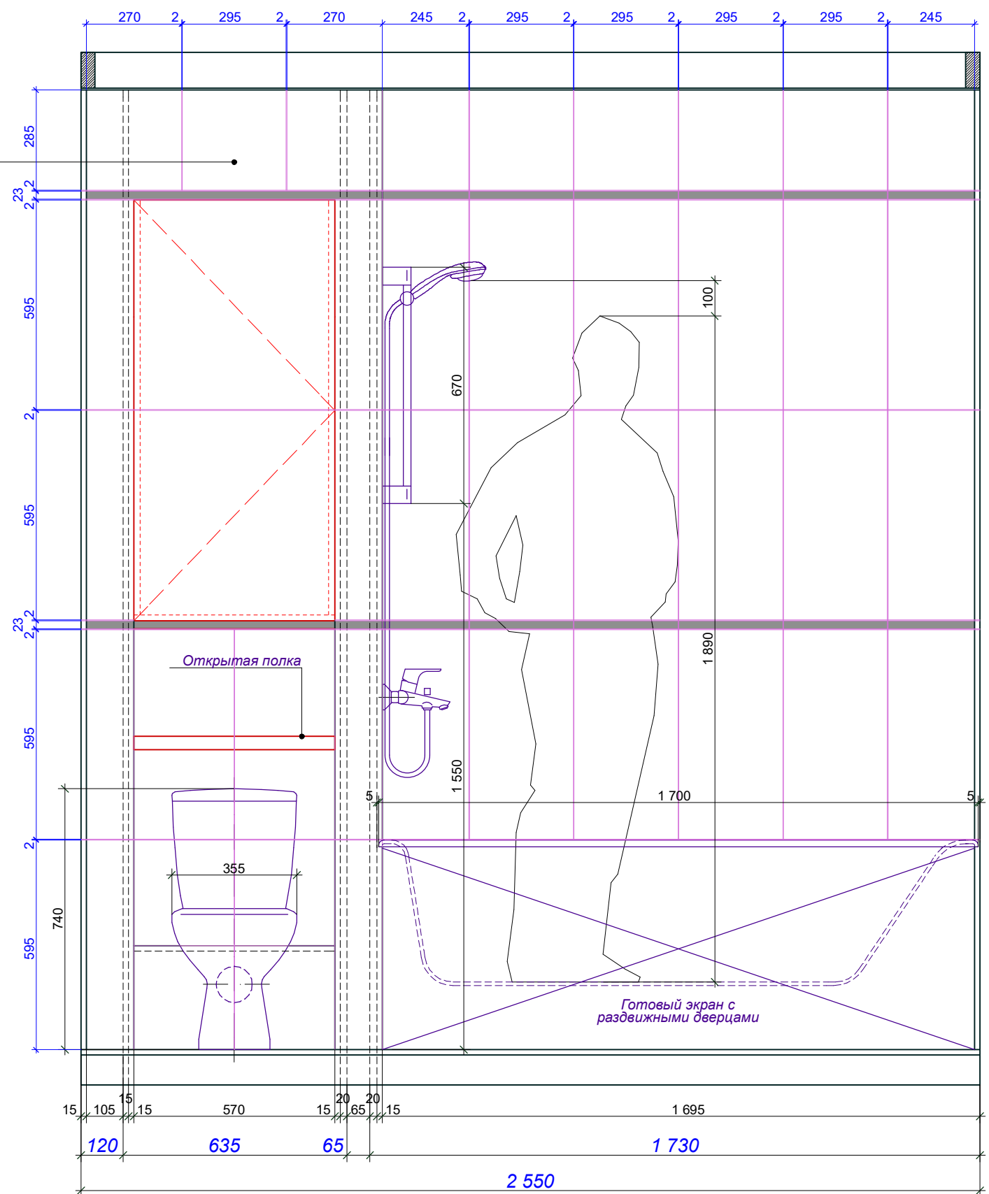
Развёртка 5
