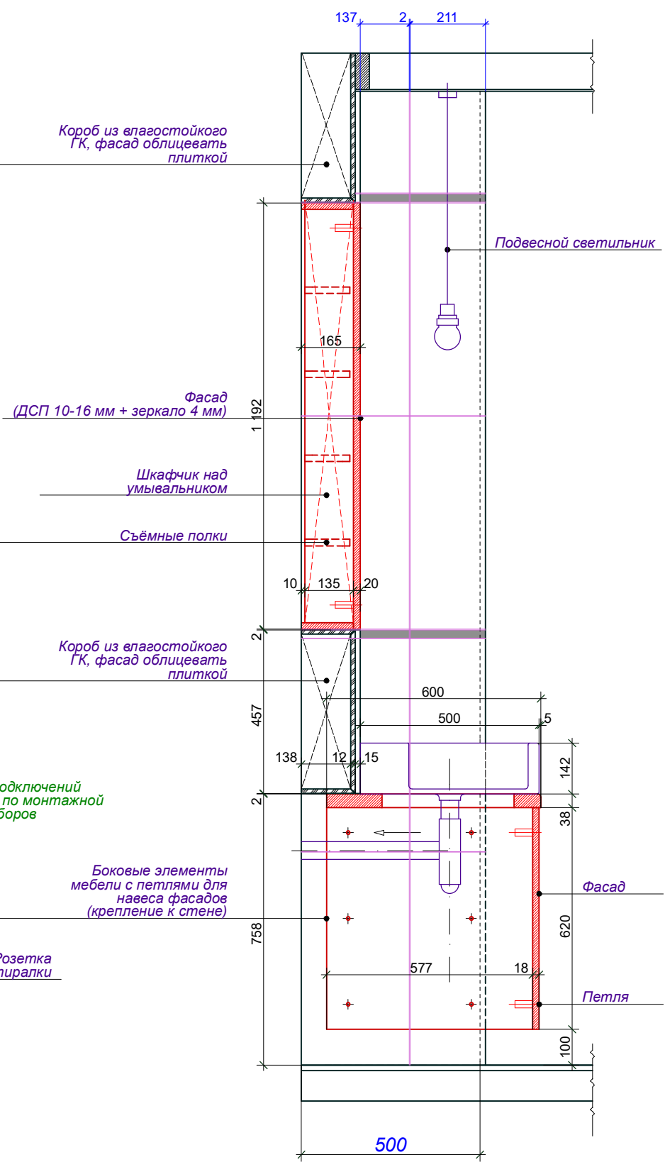
Развёртка 2
