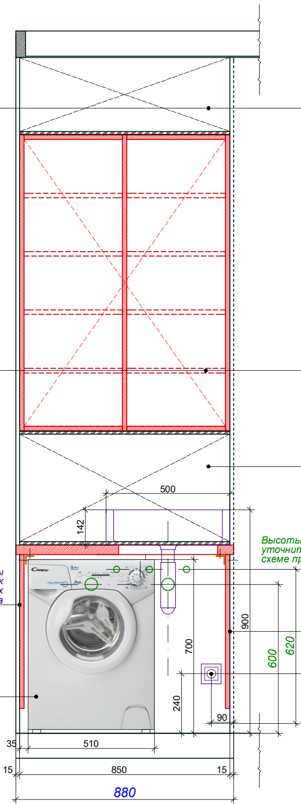
Сечение мебельного модуля по развёртке 3
