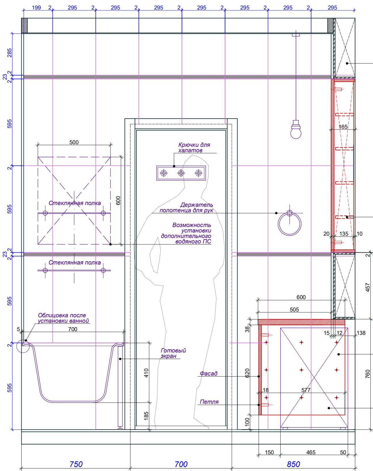
Развёртка 1
