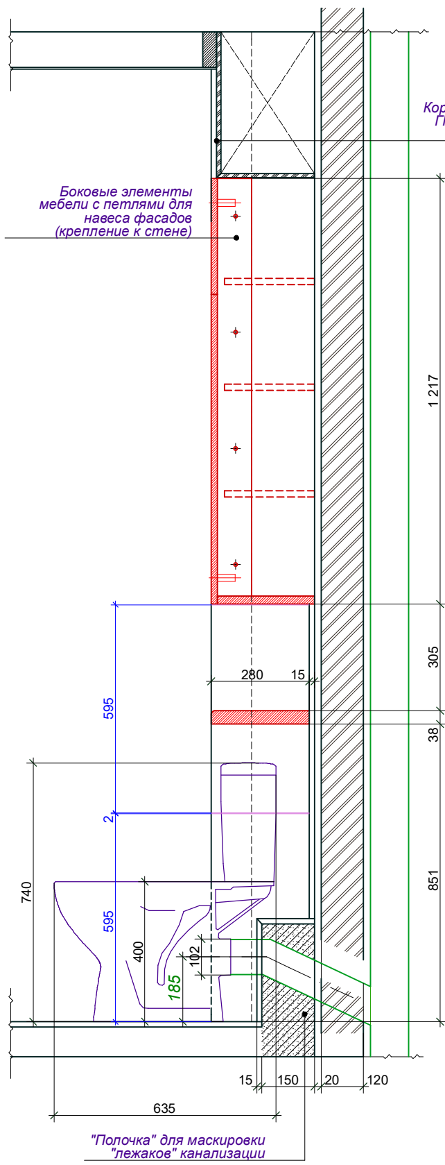
Сечение мебельного модуля по развёртке 4
