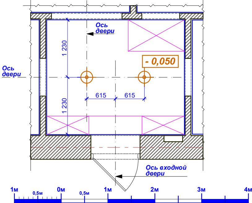
План потолка прихожей. Вариант 2а (1:50)
