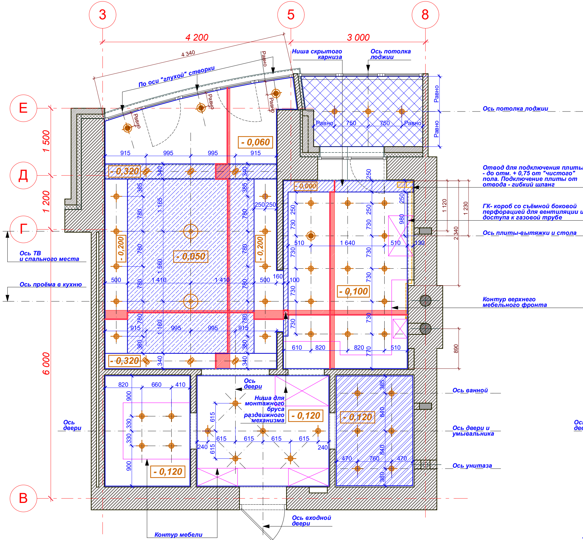
План потолка прихожей. Вариант 2а (1:50)
